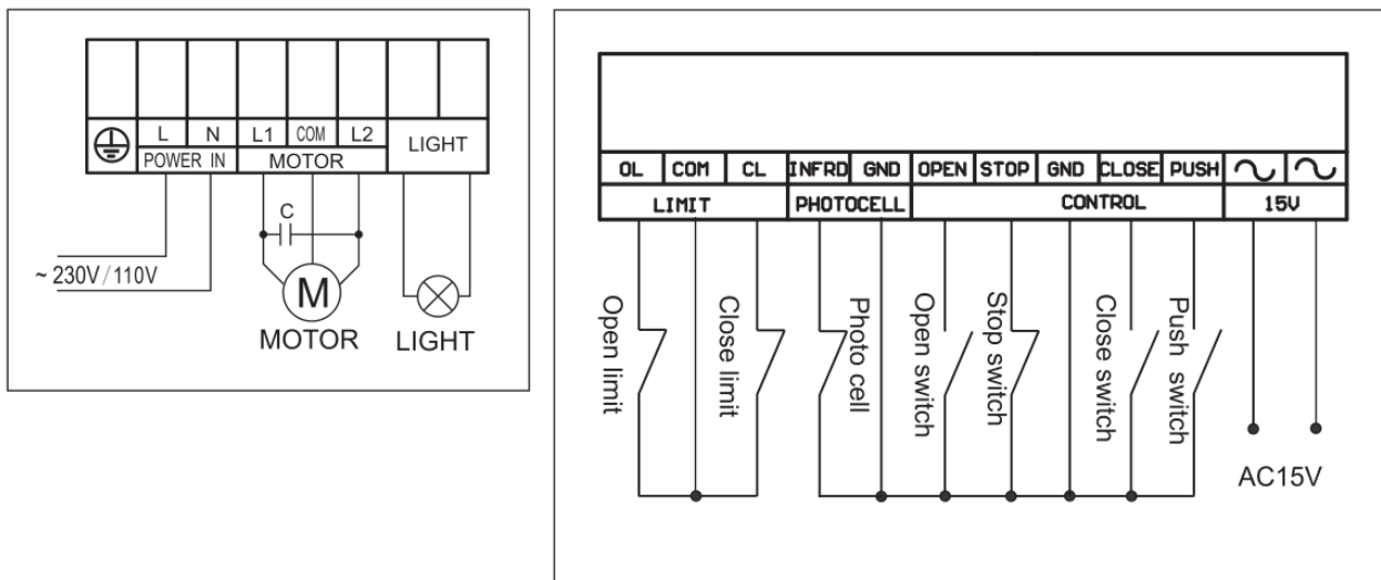
Рис.7 Схема подключения
