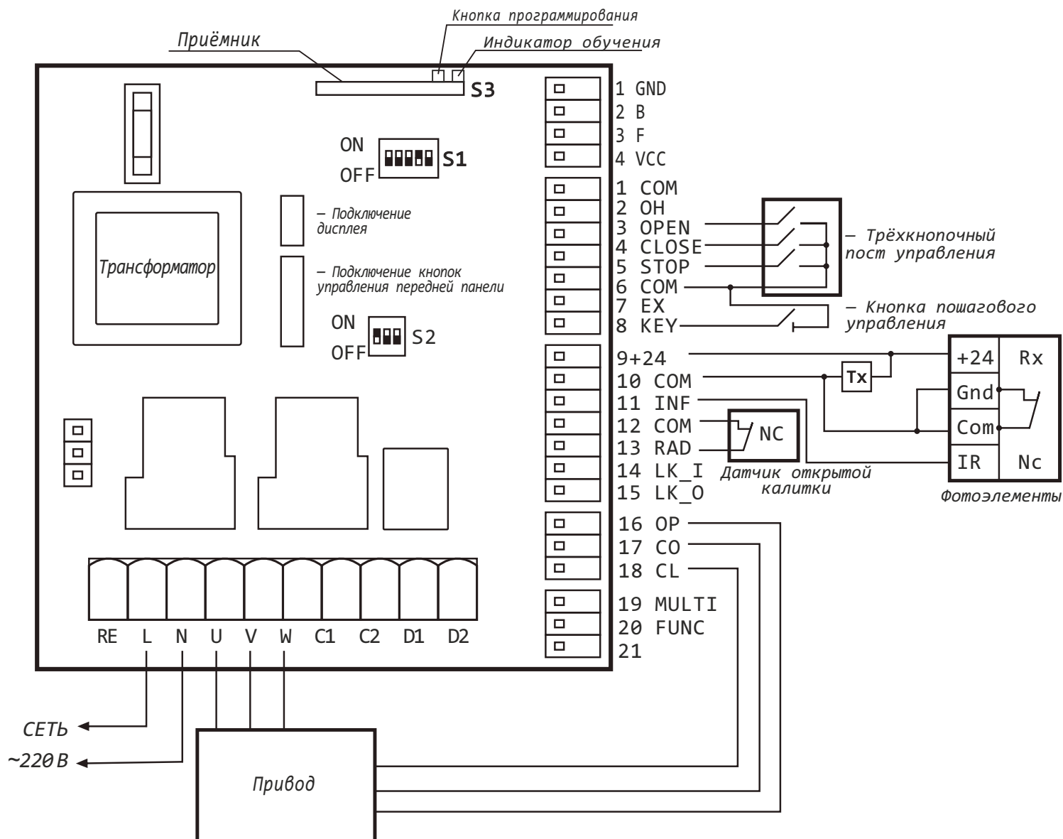
Рис. 6. Схема подключения
